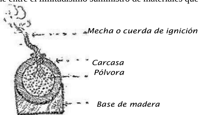
SECCIÓN DE UN OBÚS
